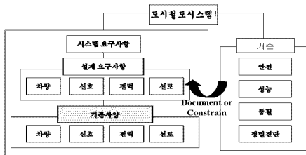
<그림 3> 시스템 요구사항의 분류
