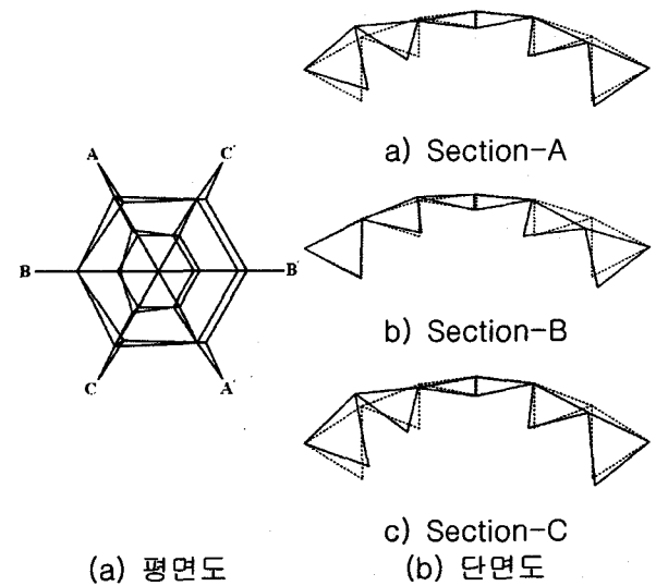
<그림 12> 가상모델 (Type-B, ×1000배)
