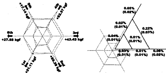
(a) 누적장력량 (b) 부재장력 오차율 <그림 18> 최종시공해석 (Case-3)
