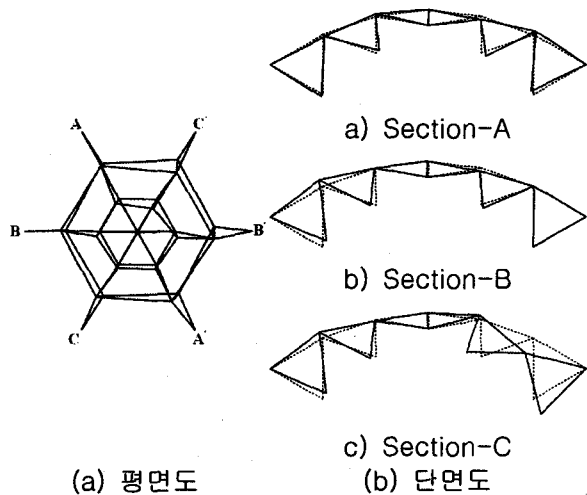
(a) 평면도 (b) 단면도 <그림 5> 가상모델 (Type-A, ×10000배)
