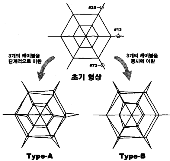
<그림 4> 가상모델의 설정
