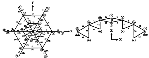
(a) 평면도 (b) 단면도 <그림 3> Geiger형 케이블 돔
