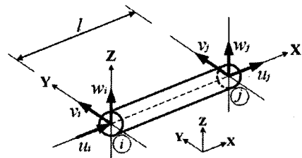
<그림 1> 케이블 요소의 요소 좌표계
