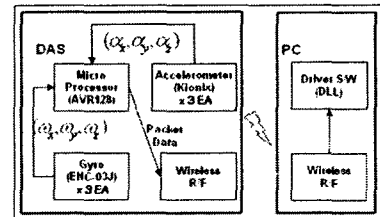
그림1. 동작 추적 장치의 블록 다이어그램
