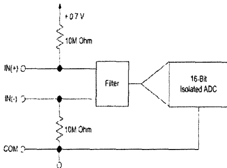
그림 4 1채널에서 아날로그 입력회로 (cFP-TC-120)
