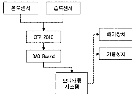
그림 1 시스템 블록도
