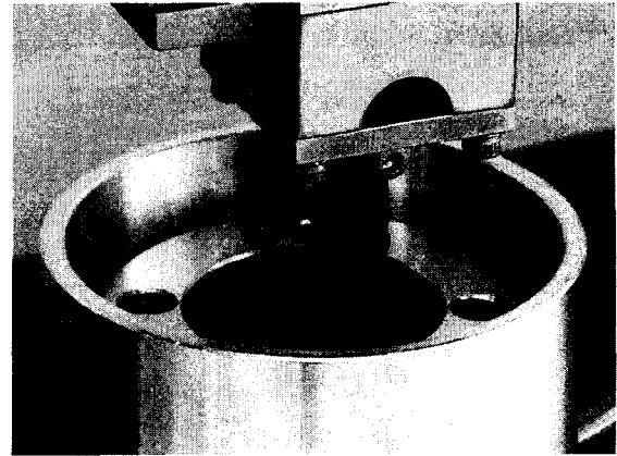
Fig. 4 Pin-on-disk type sliding test
