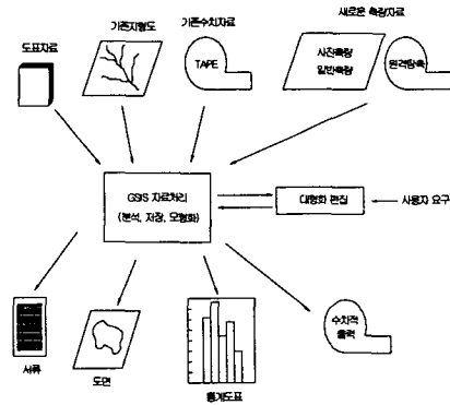
그림 1. 지형공간정보체계의 구성
