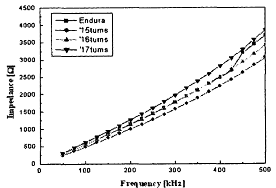
그림 4. 주파수 및 코일 권선수에 따른 임피던스 특성 Figure 4. The Impedance characteristics as a function of frequency and coil turns
