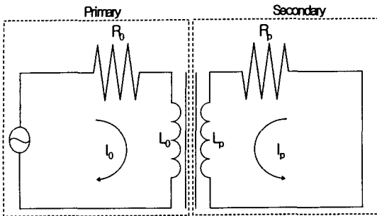
그림 1 무전극 형광램프의 전기적 등가 회로 Figure 1. Equivalent circuit of experimental circuit
