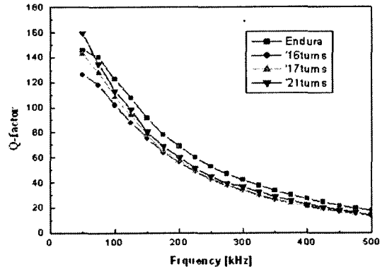
그림 3. 주파수 및 코일 권선수에 따른 Q-factor 특성 Figure 3. The Q-factor characteristics as a function of frequency and coil turns
