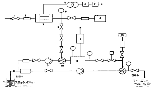
그림 4. 수산기발생장치와 처리공정도.
