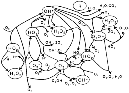
그림 1. 플라즈마 반응과정의 수산화기 발생 경로.
