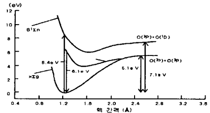
그림 2. 산소분자 에너지에 대한 전이곡선.
