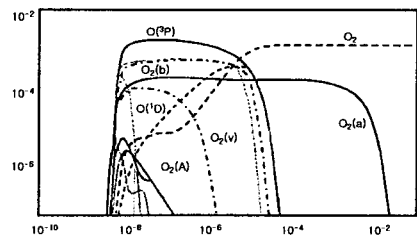
그림 3. 산소분자의 해리 과정.
