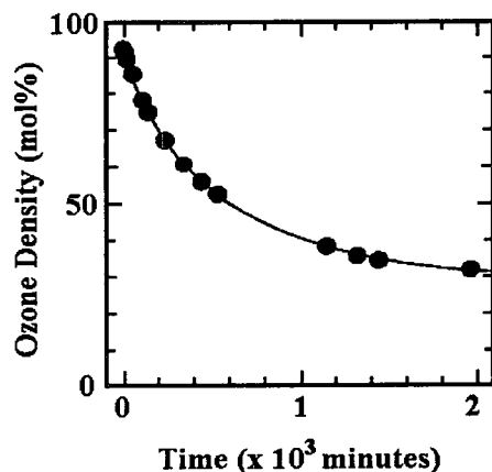
그림 3. 성막실 장치 내 오존 농도 변화.
