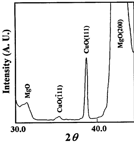
그림 4. Cu 박막의 X선 회절 패턴.
