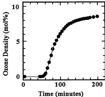
그림 2. 실리카겔 출구 오존농도.
