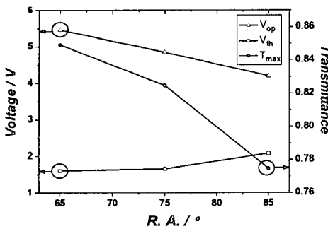
그림 3. 유전율 이방성이 양인 액정을 사용 하였을 때 러빙각에 따른 구동전압( V_{op} ), 문턱전압( V_{th} ), 최대투과율( T_{max} ) 변화를 나타내는 컴퓨터 시뮬결과.
