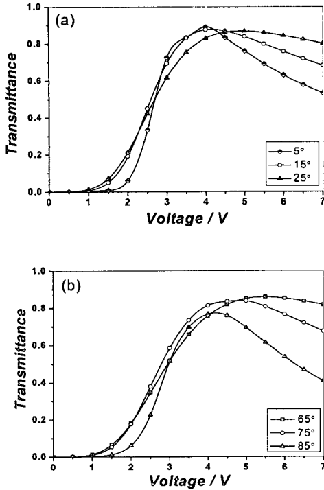
그림 2. (a) -LC 과 (b) +LC를 사용하였을 때의 전압인가에 따른 투과율.
