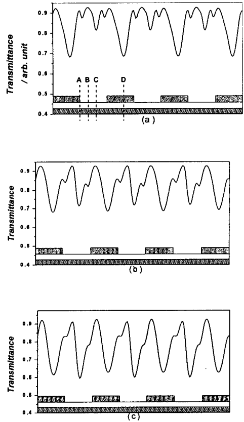
그림 4. 유전율 이방성이 양인 액정을 사용하고 러빙각이 각각 (a) a = 65^\circ , (b) a = 75^\circ , (c) a = 85^\circ 일 경우에 수평방향에 따라 발생하는 투과율을 나타내는 컴퓨터 시뮬결과.
