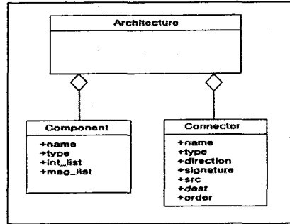
그림 4 아키텍처 명세를 위한 클래스 다이어그램
