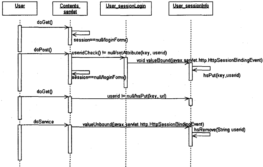
(그림 5) 접속중인 학습자를 확인 시퀀스 다이어그램
