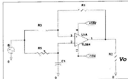
그림 5. 위상 변환기 Fig 5. phase shifter circuit
