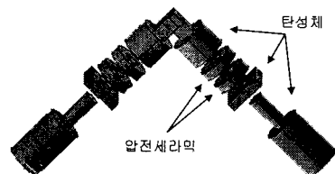
그림 1. 초음파 리니어 모터의 구조 Fig. 1. Structure of ultrasonic linear motor
