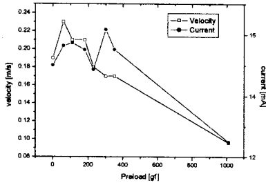
그림 6. Preload의 변화에 의한 속도와 전류 Fig. 6. Velocity and current with the change s of preload
