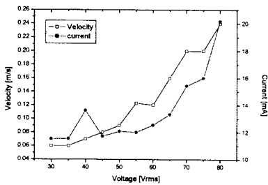
그림 7. 전압의 변화에 의한 속도와 전류 Fig. 7. Velocity and current with changes of voltage
