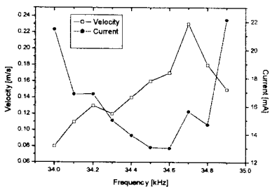
그림 8. 구동 주파수의 변화에 의한 속도와 전 류 Fig. 8. Velocity and current with the change s of driving frequency
