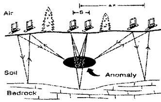
그림 1. GPR 탐사법 모식도
