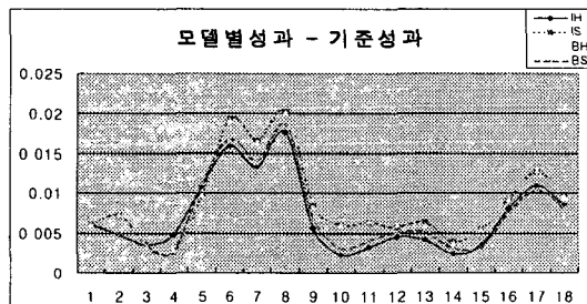
그림 8. 전리층 및 대류층 오차보정모델별 비교
