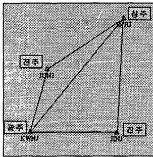
그림 4. 직삼각망 형태
