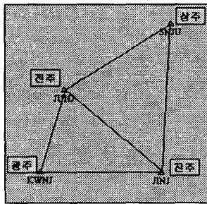
그림 3. 정삼각망 형태
