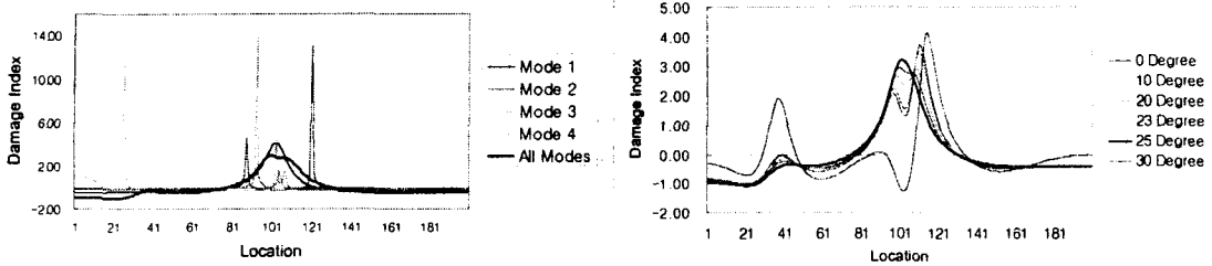
Fig. 9. 손상 고유진동수(23도) Vs 비손상 고유진동수(23도) Fig. 10. 손상 고유진동수(23도) Vs 비손상 진동수(0-30도)
