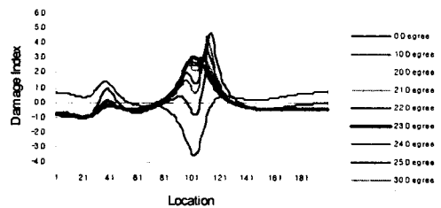
Fig. 8. 손상 고유진동수(23도) Vs 비손상 진동수(0-30도)
