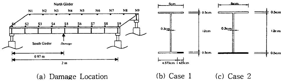
Fig. 6. 손상 위치 및 크기
