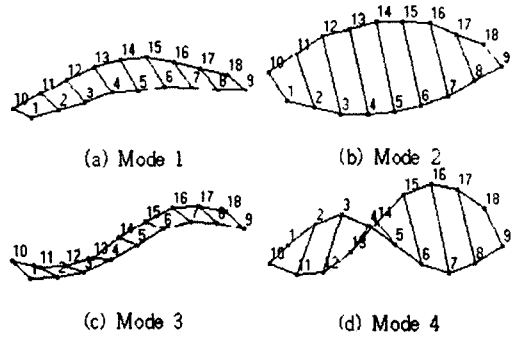
Fig. 3 강판형 모형의 모드형상
