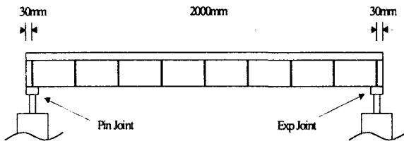
Fig. 1 강판형교 모형
