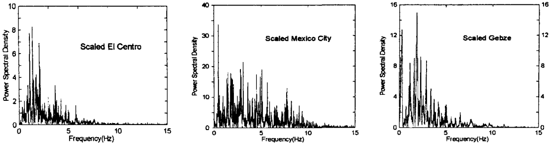
그림 4. 각 역사 지진의 Power Spectral Density
