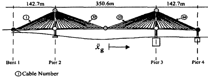
그림 2. Bill Emerson Memorial Bridge(벤치마크 사장교모델, Dyke 등, 2003)
