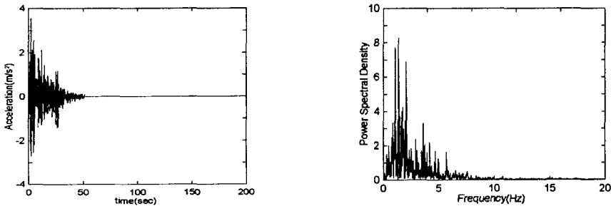
a) 가속도 시간 이력곡선
