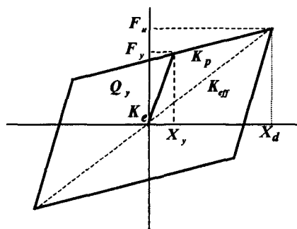
그림 1. 납고무 받침의 거동 및 설계 요소
