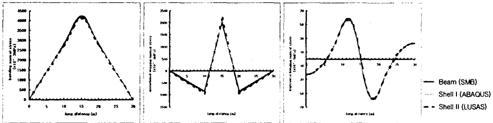
[그림7] 범요소와 쉘요소에 의한 응력 비교
