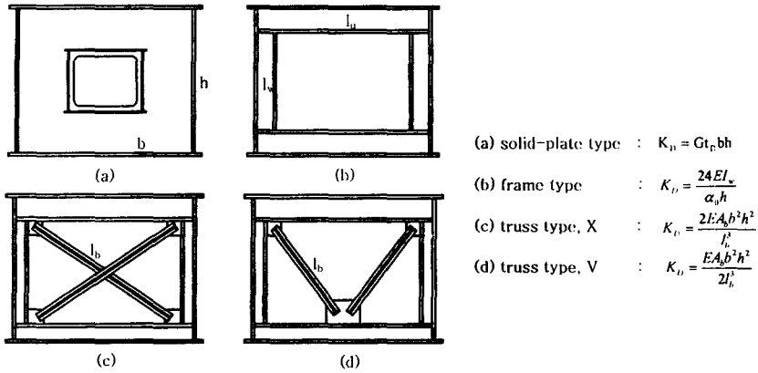
[그림4] 격벽의 종류와 강성산정식
