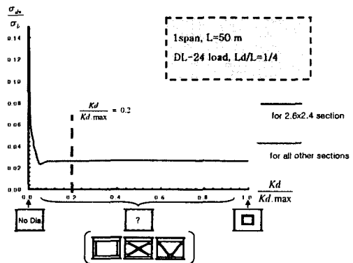
[그림9] 최소 격벽 강성비
