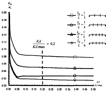
[그림13] 격벽 간격별 법선응력과 격벽강성비
