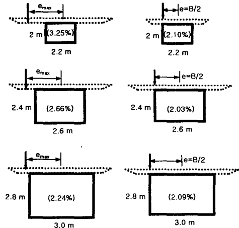
[그림12] 편심거리별 법선응력비(관호안값)
