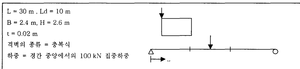
[그림6] 해석프로그램 검증 모델링 재원
