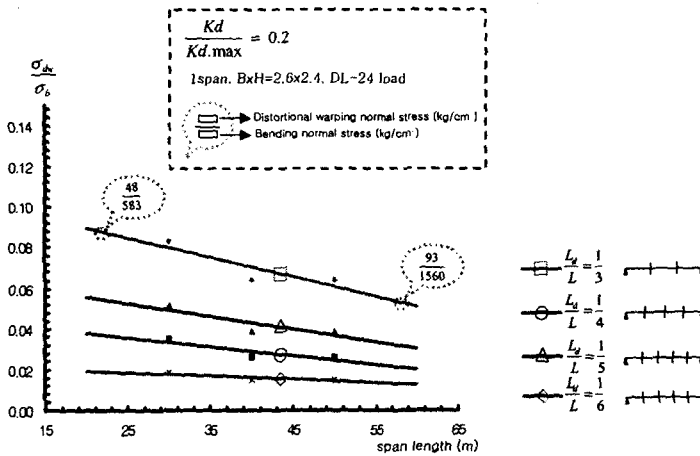
[그림 14] 단경간에서의 지간길이와 법선응력비
