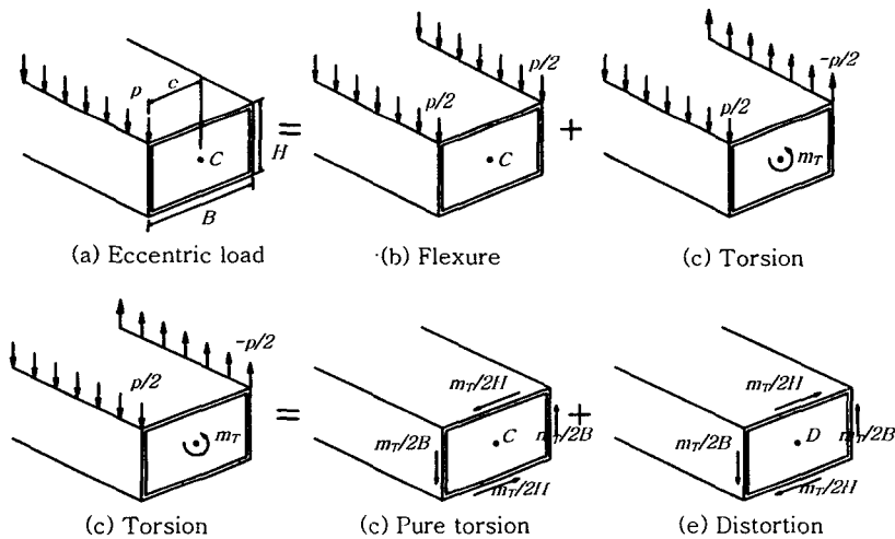
[그림1] 강상자위에 작용하는 편심하중의 분리
