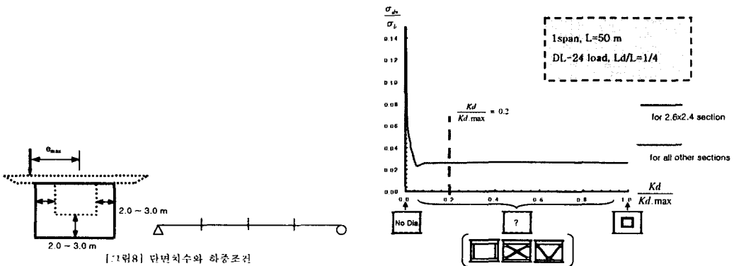
[그림9] 최소 격벽 강성비
