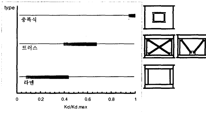
[그림5] 격벽강성비의 종류별 분포
