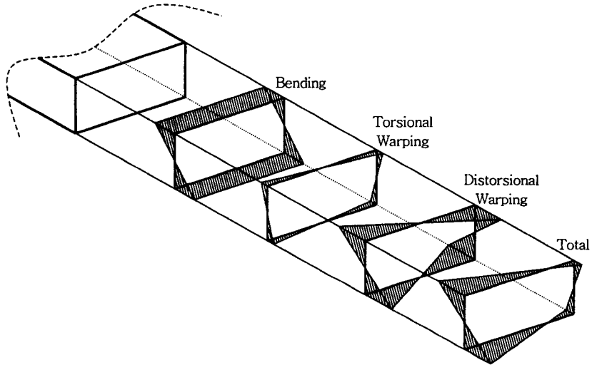
[그림2] 단실 강박스 위에 작용하는 응력성분들의 분포
