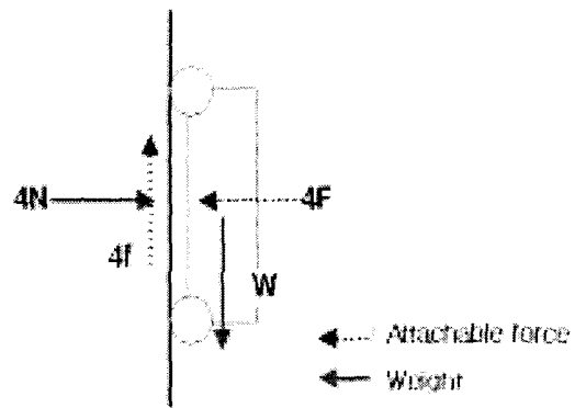
Fig. 4 weight and attachable force on vertical attaching 수직면에서 마찰력에 의한 힘을 산출하고 부착을 위해 요구되는 각 바퀴의 단위 부착력을 알기 위해서 Fig.4의 상대에 대해서 Fig.5의 3 차원 그래프를 그려보는 것이 유효하다.
