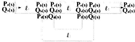
Fig. 2 Hydraulic pipeline with a parallel line. 위 식에서 식의 표기를 간단히 하기 위하여 \sinh(\Gamma_i) , \cosh(\Gamma_i) , Z_{ci} 를 각각 S_i , C_i , Z_i 로 표기하였으며 i 는 관로번호를 나타낸다. 동일한 방법으로 계산하여 얻어진 병렬 유압관로의 입구와 출구 사이의 유동 관계식은 다음과 같다.
