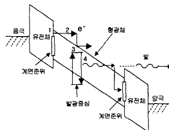
그림 1. 에너지 밴드도
