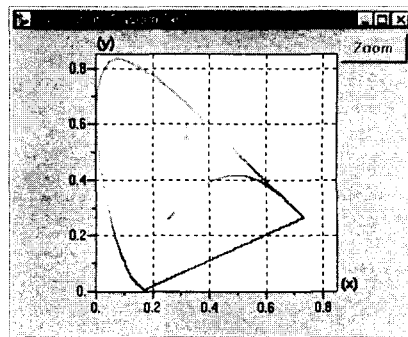
그림 8. 고휘도의 색좌표
