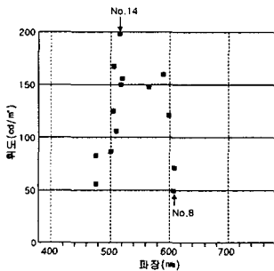
그림 12. 파장에 따른 휘도 분석
