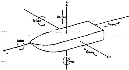
Fig. 1 . 선박의 6자유도 운동
