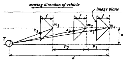
그림 8. 망원카메라를 이용한 표지판의 위치예측
