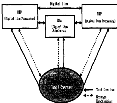
그림 1. DIP, DIA, 툴 서버와의 관계
