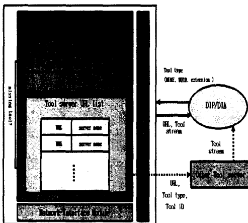
그림 2. 툴 서버 구조도
