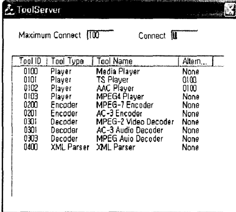
그림 5. 툴 서버의 AAC.player 검색
