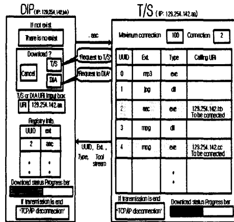
그림 3. 툴 서버와 DIP의 툴 전송 시나리오의 예
