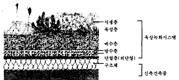
그림 2. 신축건축물 옥상녹화 하부시스템 구성
