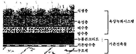
그림 1. 기존 건축물 옥상녹화 하부시스템 구성
