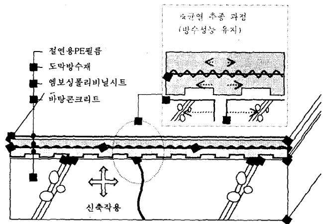
그림 6. 균열 추종 성능(방수성능 유지)
