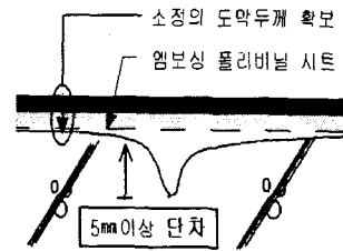
그림 10. 도막두께 확보 개념
