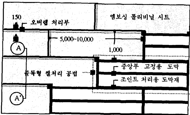
그림 9. 절연접착 평면도
