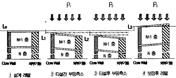
그림 1. 슬래브 타설 전후의 축소량
