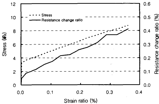
그림 9. 모르터 시험체의 변형에 따른 응력·저항변화율 곡선
