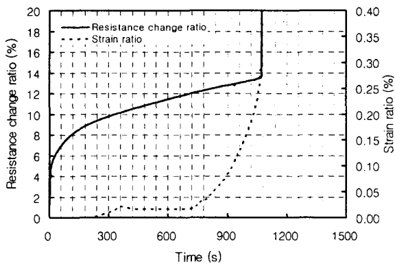
그림 10. CPGFRP를 적용한 콘크리트 시험체의 시간경과에 따른 응력·변형·저항변화율 곡선
