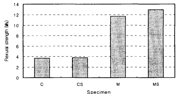
그림 6. 모르타르 및 콘크리트 시험체의 휨강도
