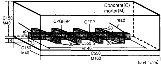
그림 5. CPGFRP 복합체를 적용한 시험편의 모식도
