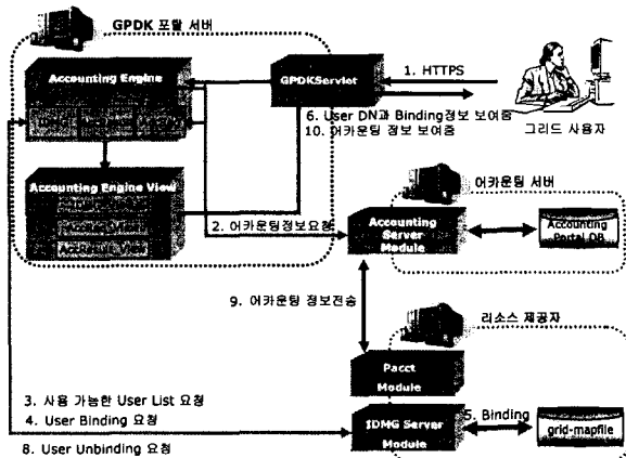
그림5 GPDK를 이용한 그리드 어카운팅 포탈 구조
