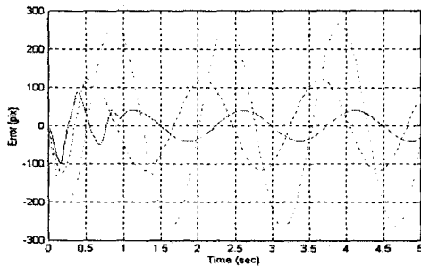
(- · - : 비례 제어기, - - - : PID 제어기, — : 극배치 제어기)
