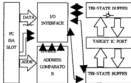
그림 1. 전체 BLOCK DIAGRAM
