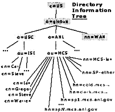
<그림 2> 디렉토리 정보 트리의 예
