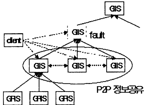
<그림 3> P2P 기반 정보 서비스
