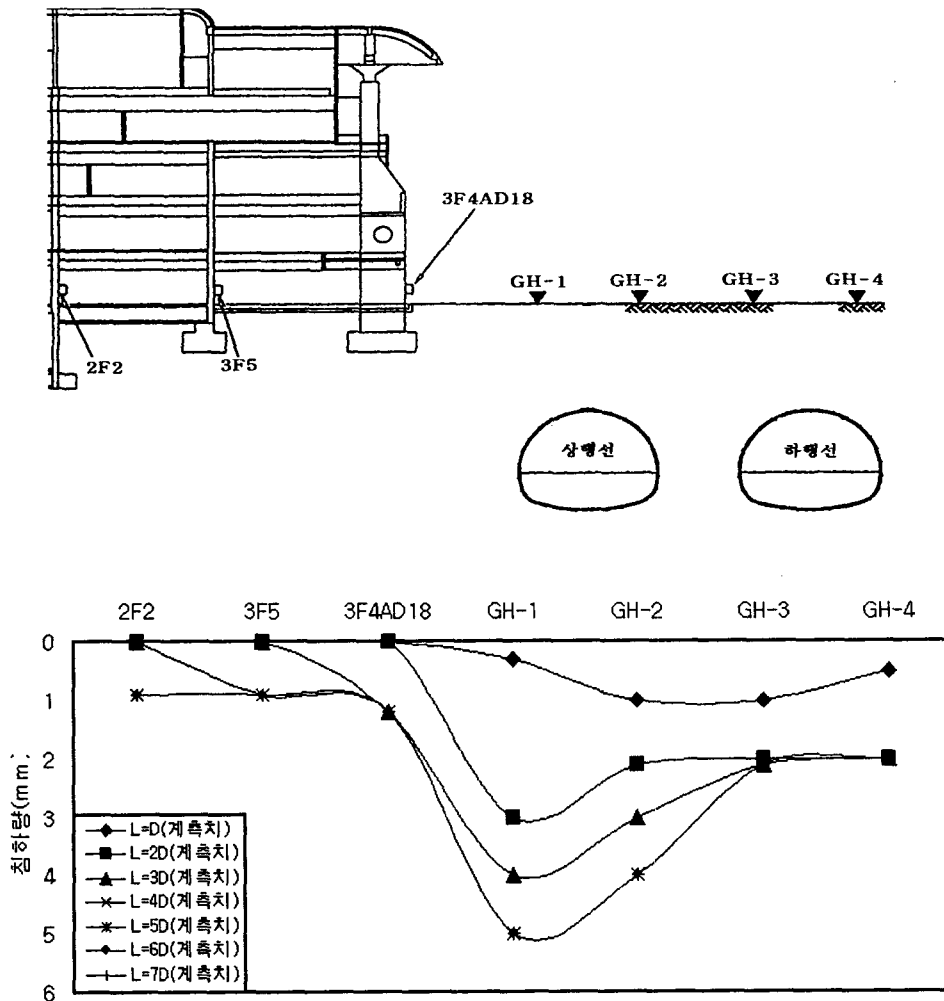
그림 8. 막장진행에 따른 지반 및 구조물의 거동
