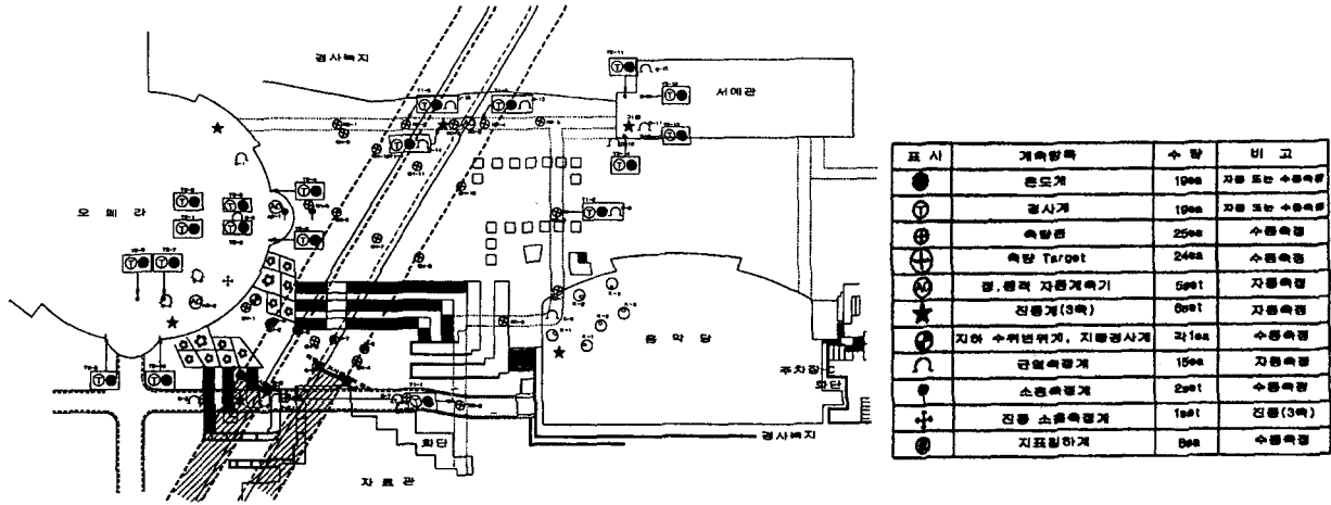
그림 3. 현장 계측기설치 평면도
