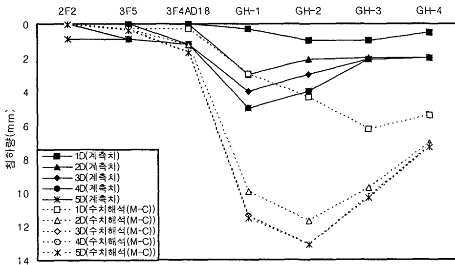
그림 9. 계측치와 수치해석에 의한 지반 및 구조물
