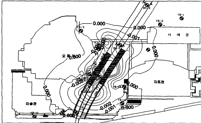
그림 6. 지반 및 구조물의 침하영향 변화
