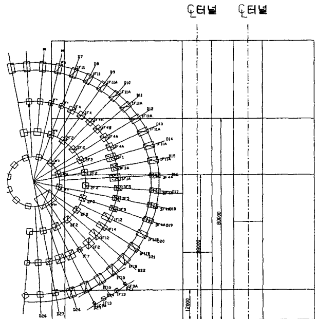
그림 5. 건물 기초의 위치평면도
