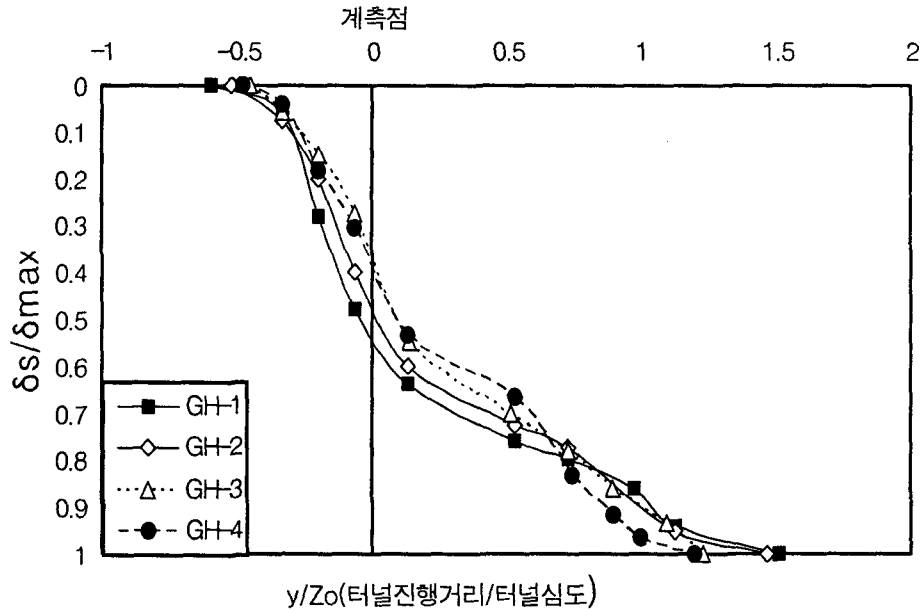
그림 7. 종방향 지표침하 영향거리
