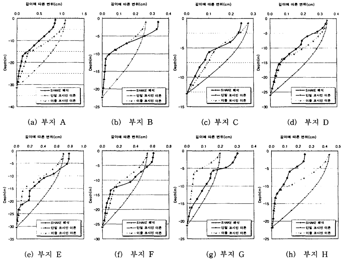
그림 7 지진응답해석 결과와 단일·이중코사인법으로 구한 지중변위 비교(내진 1등급 지진재해도 재현주기 1,000년 이용)
