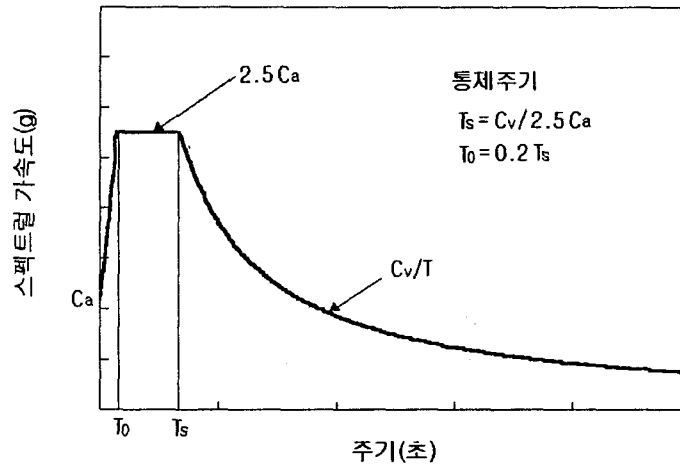
그림 2 지표면 표준 설계응답스펙트럼 (건설교통부, 1997)
