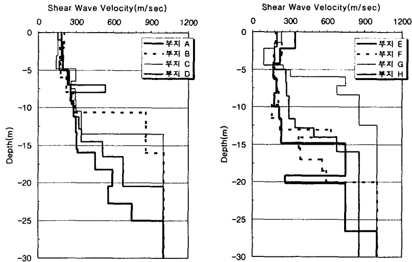
그림 3 해석대상 지반의 전단파속도 주상도
