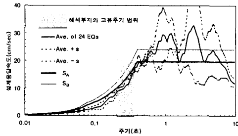
(b) 행정구역 기준 이용
