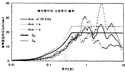
(a) 지진재해도를 이용(재현주기 1,000년)
