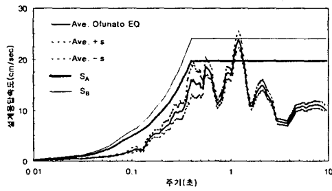
(a) Ofunato 지진파 이용 결과
