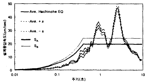
(b) Hachinohe 지진파 이용 결과
