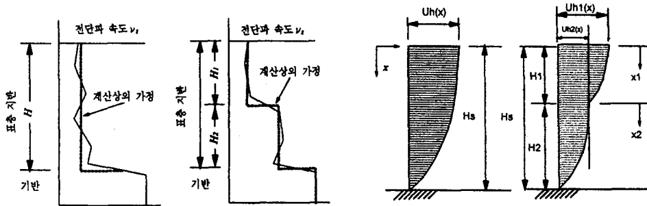
(a) 지층의 분할 및 평균 전단파속도 산정
