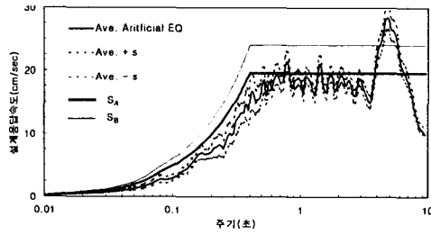
(c) 인공지진과 이용 결과
