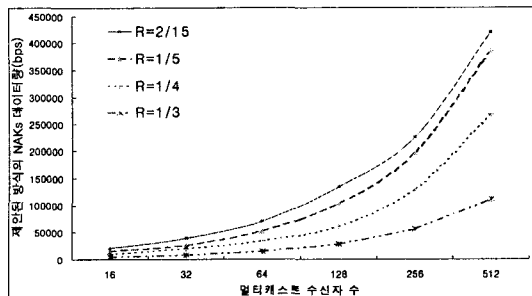
그라프 2 제안된 방식에서 멀티캐스트 트리 전체에 전송되는 NAKs 데이터의 총합
