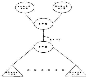
그림 3 PGM과 제안된 방식의 대역폭 소모 시뮬레이션 토폴로지
