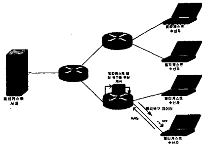
그림 2 제안된 방식에 의한 멀티캐스트 에러 복구 개념도
