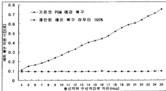
그림 3 기존 PGM과 제안된 에러 복구 방식(에러 복구 라우터의 수/라우터의 수=1)의 에러 복구 지연 시간 비교
