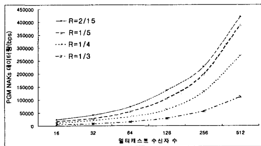
그라프 1 기존 PGM에서 멀티캐스트 트리 전체에 전송되는 NAKs 데이터의 총합
