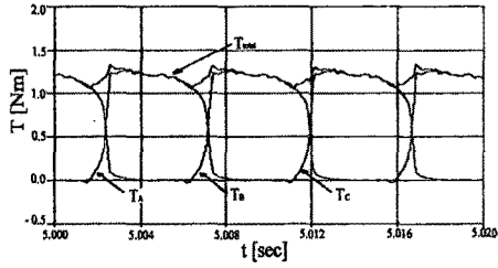
b) 정속 구간 토크 파형
