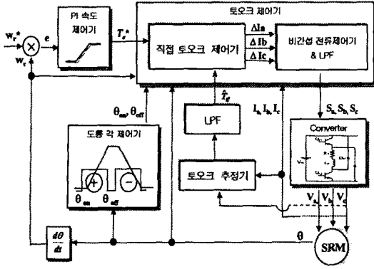
그림 1 토크 제어형 SRM 가변속 제어기
