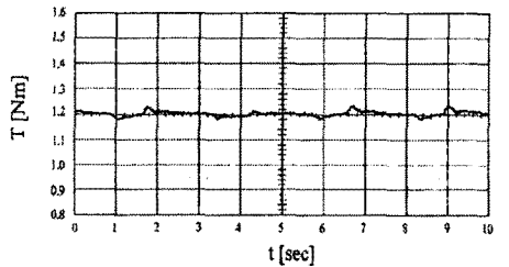
b) 정속 구간 토크 파형
