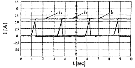
a) 정속 구간 전류
