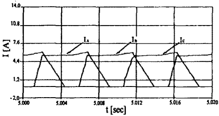
a) 정속 구간 전류 파형
