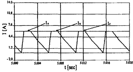
a) 정속 구간 전류 파형
