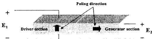
그림 1. 압전 변환기의 구조
