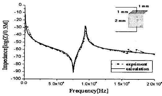
그림 2. 임피던스 파형의 비교
