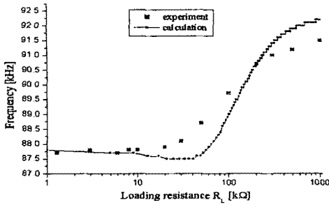
그림 7. 부하의 변화에 따른 공진 주파수의 변화
