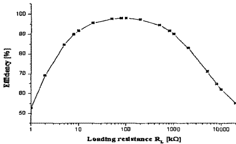
그림 9. 부하의 변화에 따른 효율의 변화
