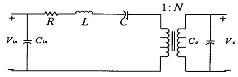
그림 6. 무부하시 압전 변압기의 등가회로
