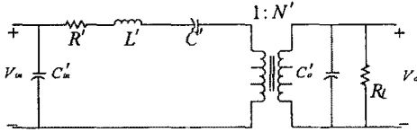
그림 8. 부하시 압전 변압기의 등가 회로
