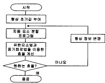
그림 4. 자동 요소분할 프로그램을 적용한 진화알고리즘의 순서도
