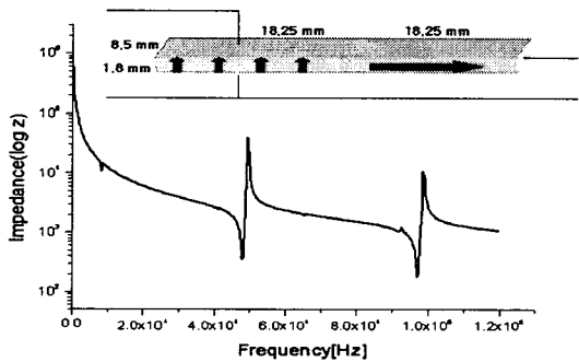
그림 3. 압전 변압기 구동부의 임피던스
