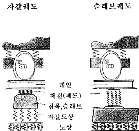
그림3. 자갈궤도 및 슬래브궤도의 시스템구성
