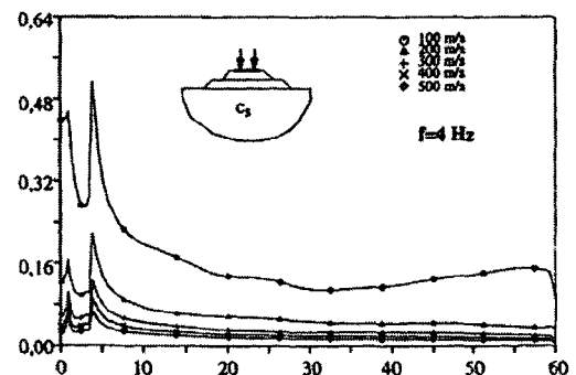
그림8. 지반특성에 따른 케도진동 및 파전달
