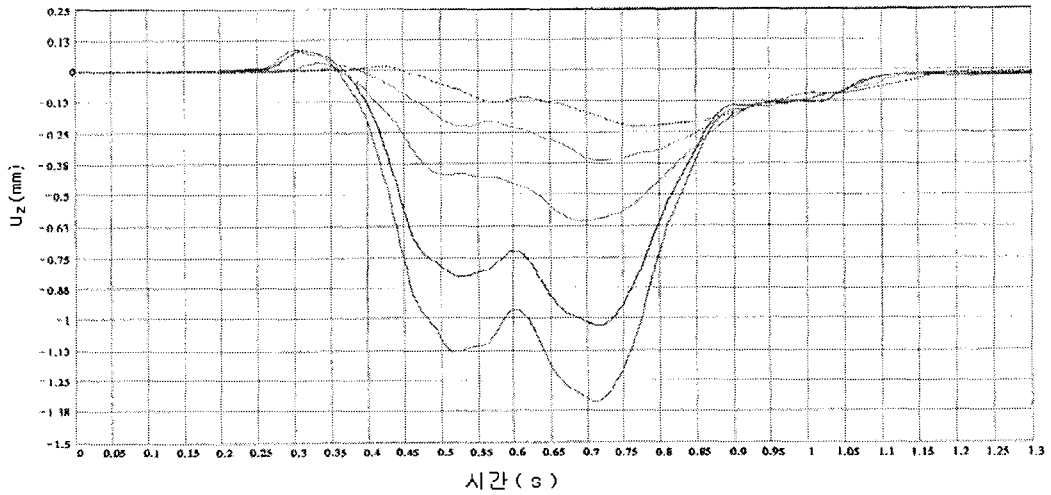
그림 13. 시간에 대한 y방향 변위(궤도의 수직변위)
