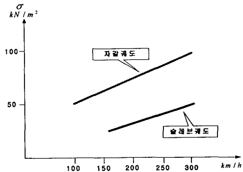
그림4. 열차속도에 따른 지반응력
