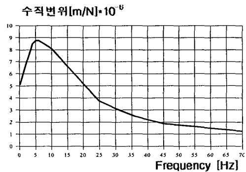
그림11. Frequency에 대한 수직변위
