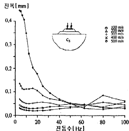
그림7. 지반특성에 따른 자갈케도의 수직변위변화
