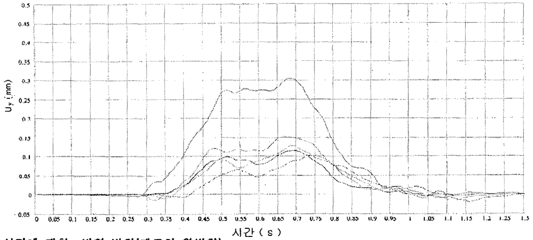
그림 12. 시간에 대한 y방향 변위(궤도의 횡방향)
