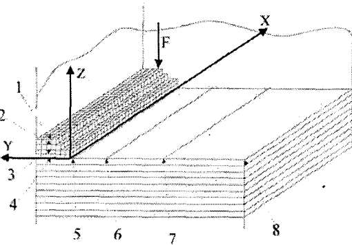
그림9. 슬래브궤도 및 지반의 모델
