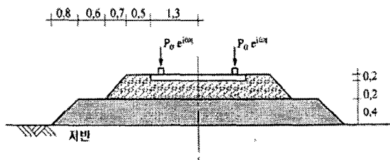
그림6. 기존자갈케도의 계산모델
