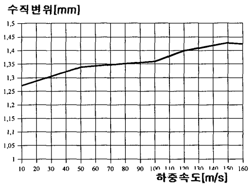
그림10. 하중속도에 대한 수직변위의 변화
