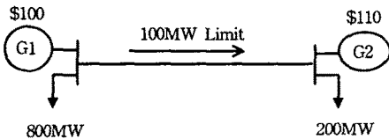
(그림 1) 2모선 사례계통 (발전기 용량제약은 없으며, 발전기 상단의 가격은 입찰가격임)
