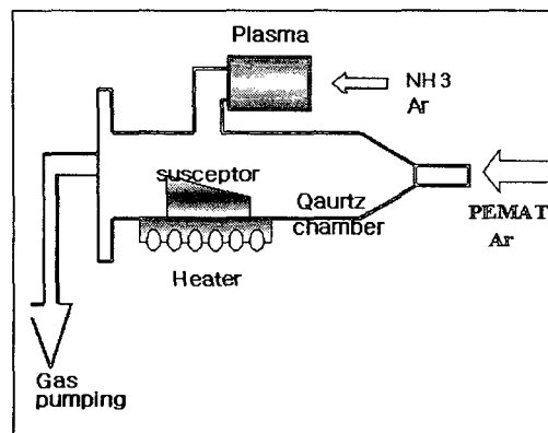
그림2. ALD chamber
