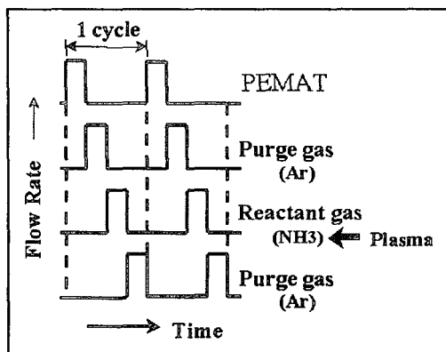
그림1. ALD 가스주입
