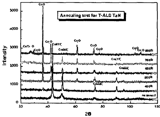
그림 5. 구리 열처리 결과에 따른 XRD 측정
