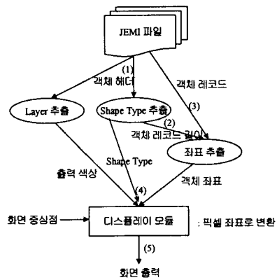
<그림 5> 객체 출력 방법
