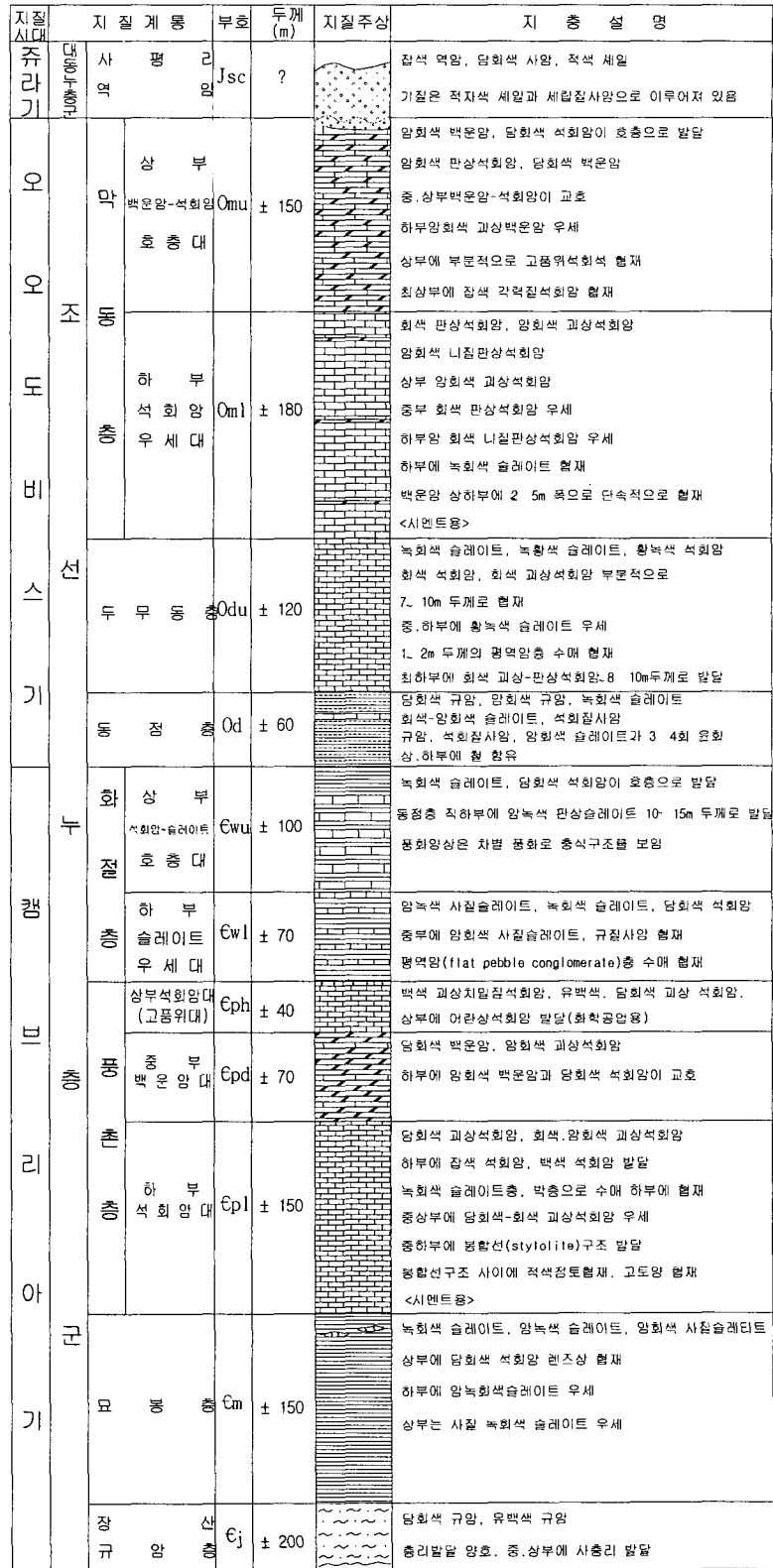
그림 2. 조사지역의 종합지질주상단면도
