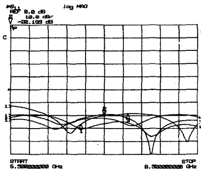
그림 9. 추적 신호블록의 입력반사손실(측정)
