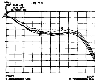
그림 2. 주 신호블록의 선형이득특성(측정)
