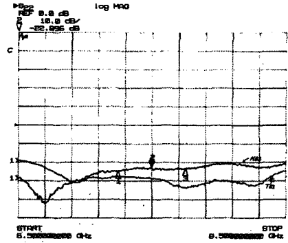
그림 10. 추적 신호블록의 출력반사손실(측정)
