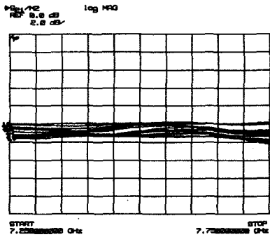
그림 8. 추적 신호블록의 위상제어에 따른 이득변화량 (측정)
