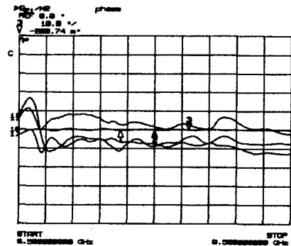
그림 6. 추적 신호블록의 채널간 초기위상오차(측정)
