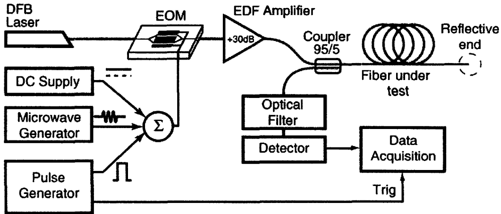
<그림-1> 산란형 광섬유를 이용한 계측시스템( BOTDR system )
