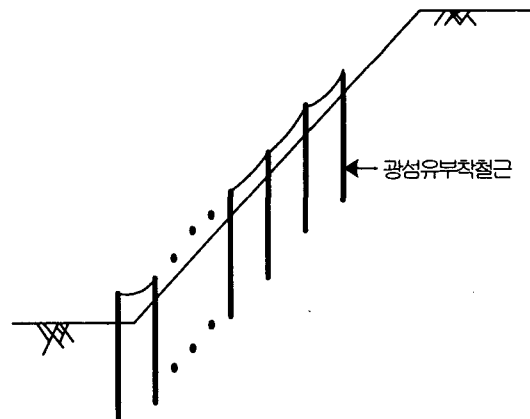
<그림-8> 광섬유 계측기의 사면 현장 설치
