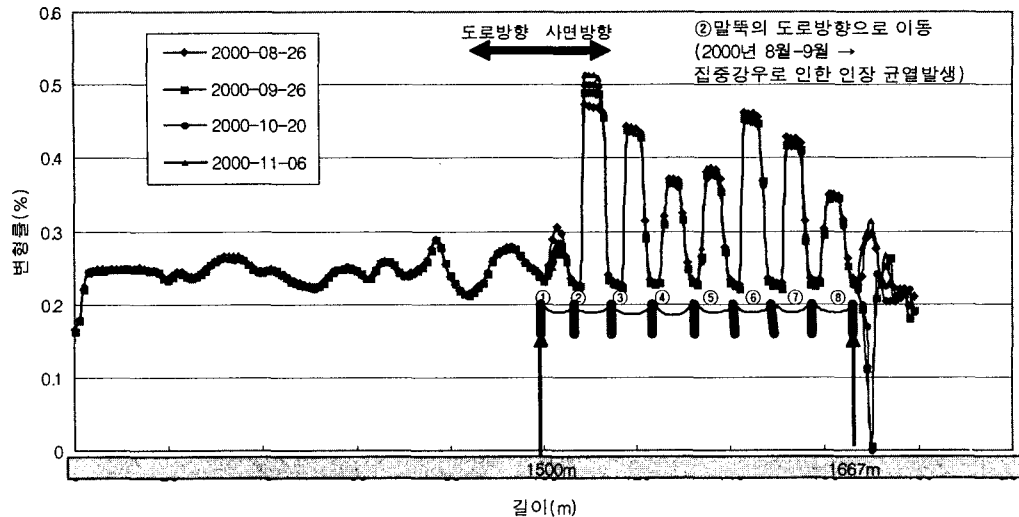
<그림-9> 산란파를 이용한 광센서(BOTDR) 계측 결과
