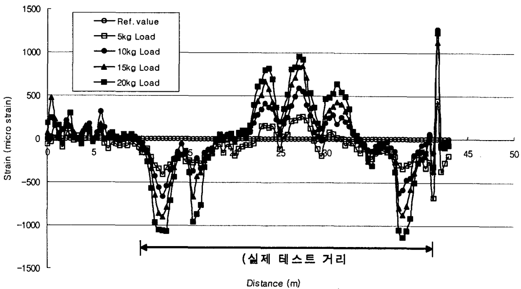
<그림-6> 산란파를 이용한 광센서 계측
