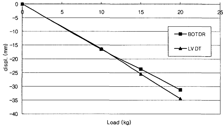
<그림-7> 측정 센서 비교
