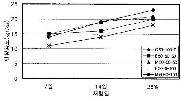
그림 10. W/C 50% 인장강도 실험결과
