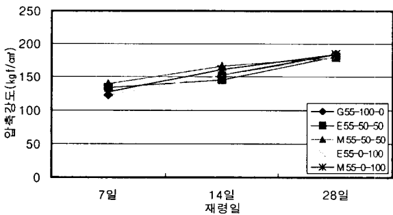
그림 9. W/C 55% 압축강도 실험결과
