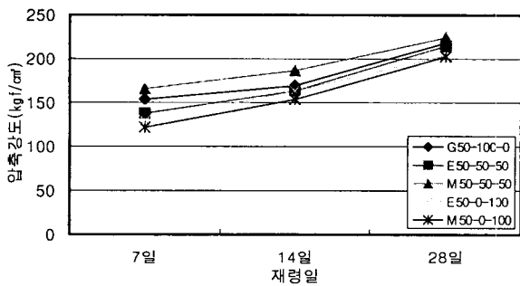
그림 8. W/C 50% 압축강도 실험결과
