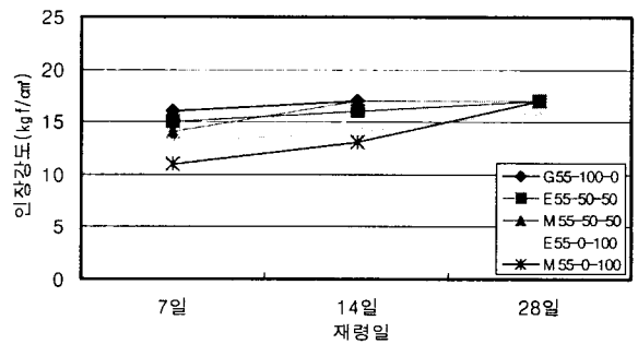
그림 11. W/C 55% 인장강도 실험결과
