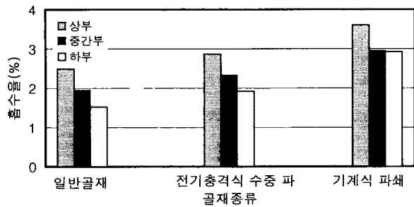
그림 12. 모의 시험체 흡수율 실험결과
