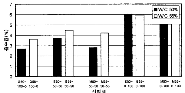
그림 7. 흡수율 실험결과
