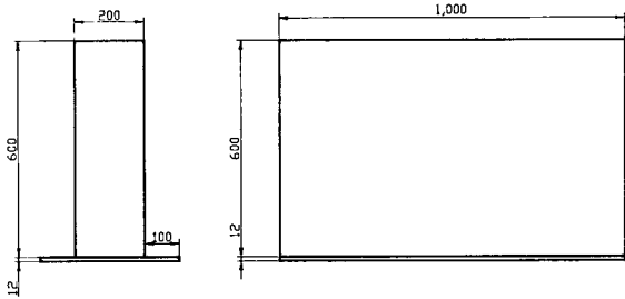
그림 3. 거푸집 입면
