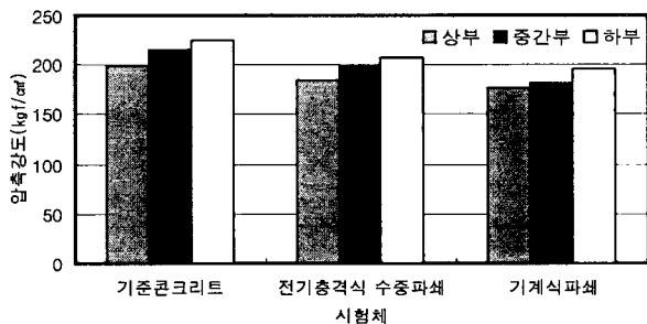
그림 13. 모의 시험체 압축강도 실험결과
