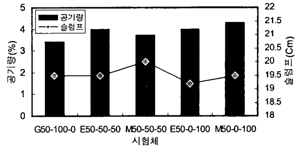
그림 5. W/C 50% 슬럼프 및 공기량 실험결과
