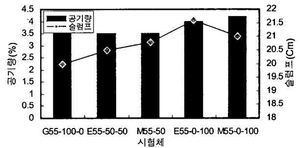
그림 6. W/C 55% 슬럼프 및 공기량 실험결과
