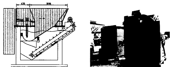
그림 1. 전기충격식 수중파쇄 시스템
