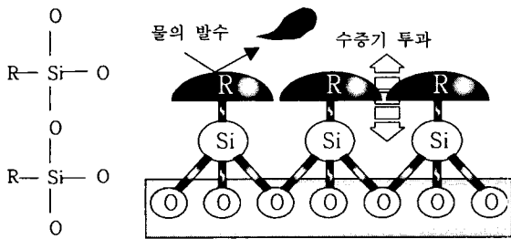
그림 2. 무기질 흡수방지제의 화학적 구성과 발수 메카니즘
