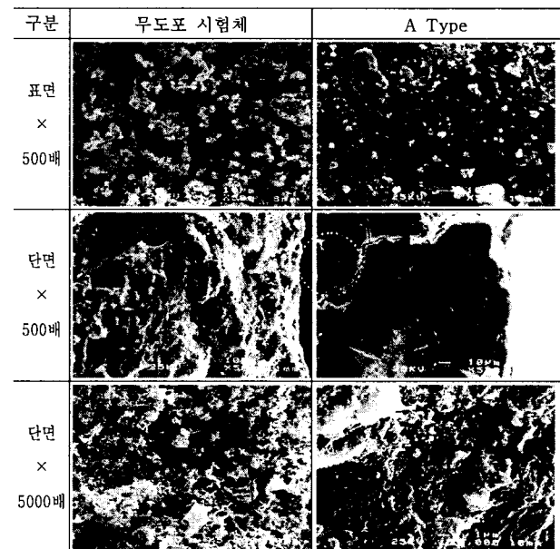
사진 5. SEM 관찰 결과
