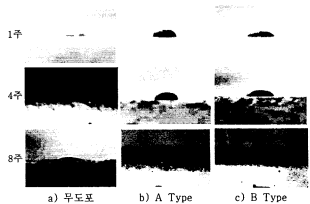
사진 4. 흡수방지재 도포에 따른 재령별 잉크의 발수성상
