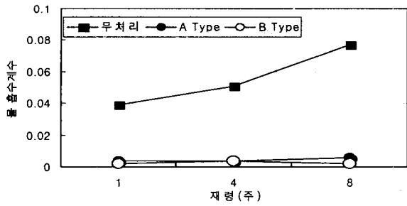
그림 5. 흡수시험 결과
