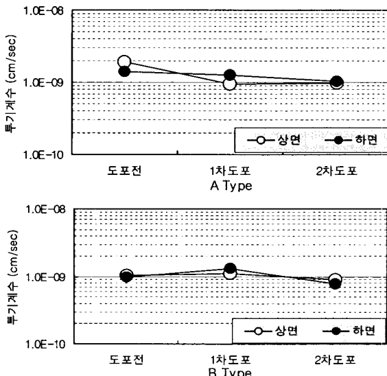
그림 6. 흡수방지재 도포 시험체의 투기계수 측정결과
