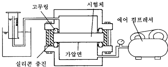
그림 3. 투기 시험 장치
