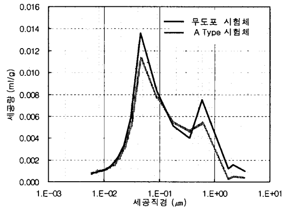
그림 7. 무처리 시험체 및 A Type 흡수방지재 도포 시험체의 세공경 측정결과
