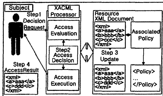
[ 그림 1 ] XACML 프로세스 개념도
