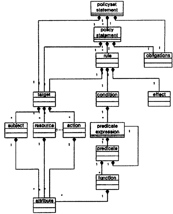
[그림 2] 정책 언어 모델
