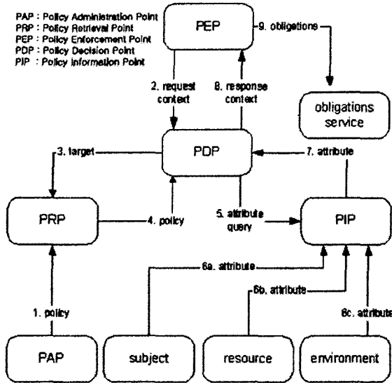
[그림 3] 데이터 흐름 모델
