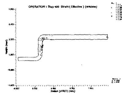
(d) Strain deformation of 4th-drawing
