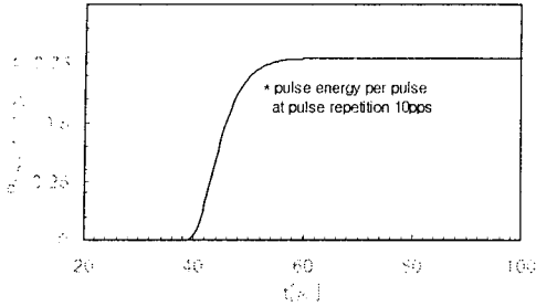
(b) 펄스코로나 방전동안의 펄스에너지 그림 6 펄스코로나 방전동안의 임피던스 및 펄스에너지 변화 특성 Fig. 6 Characteristics of impedance and pulse energy during puls corona discharging
