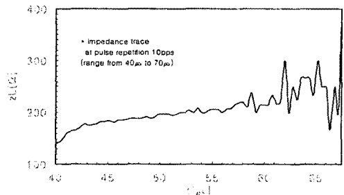
(a) 방전시간동안의 임피던스 변화곡선
