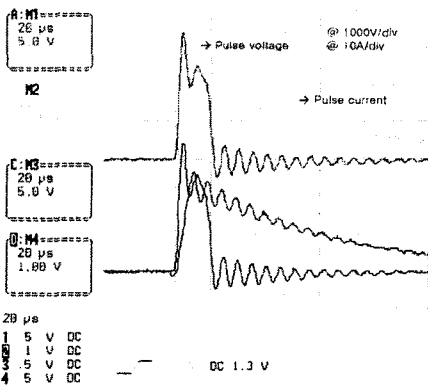
그림 3 정극성, 부극성의 펄스전압 및 전류파형 비교 Fig. 3 Pulse voltage and current waveforms of positive, negative
