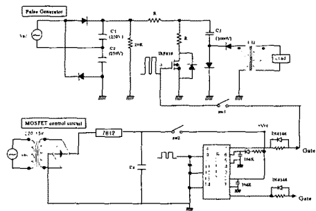
그림 1 펄스발생회로 및 MOSFET 제어회로 Fig. 1 Schematic of pulse generator and MOSFET control circuit
