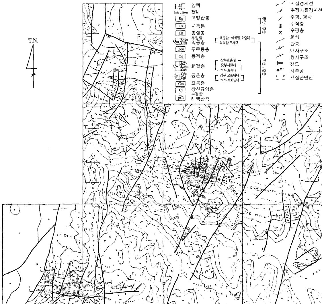
그림 1. 삼척-도계지구 지질도
