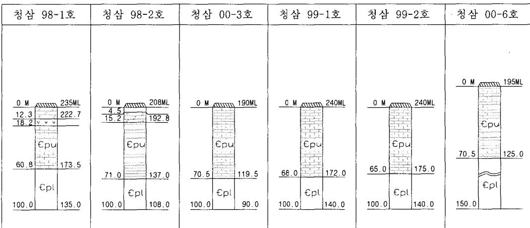
그림 7. 삼척-도계지구의 시추탐사결과 확인된 풍촌층 석회석의 부존심도
