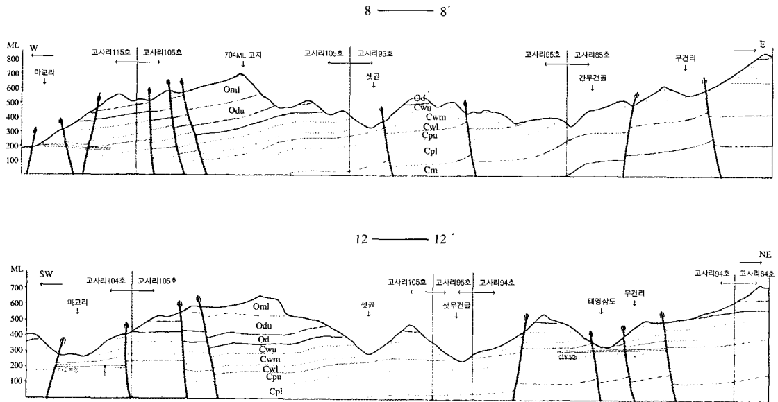
그림 2. 지질단면도
